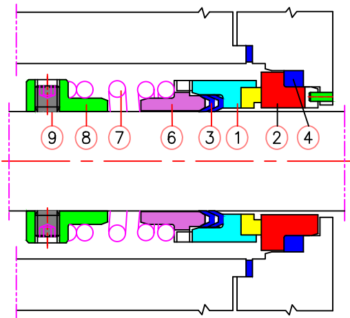
Type 8221
